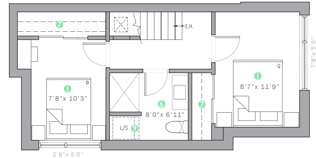
NIVEAU 0 - 436 PI.CA
