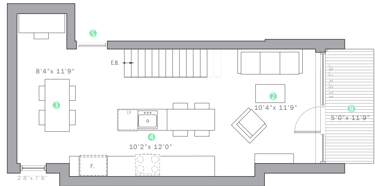
NIVEAU 2 - 475 PI.CA
