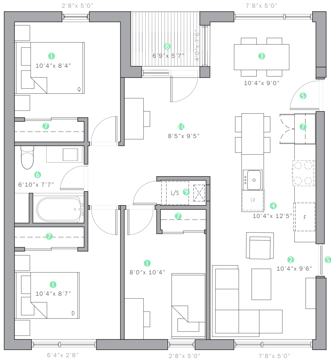
NIVEAU 1 (OPTION 1) - 996 PL.CA
