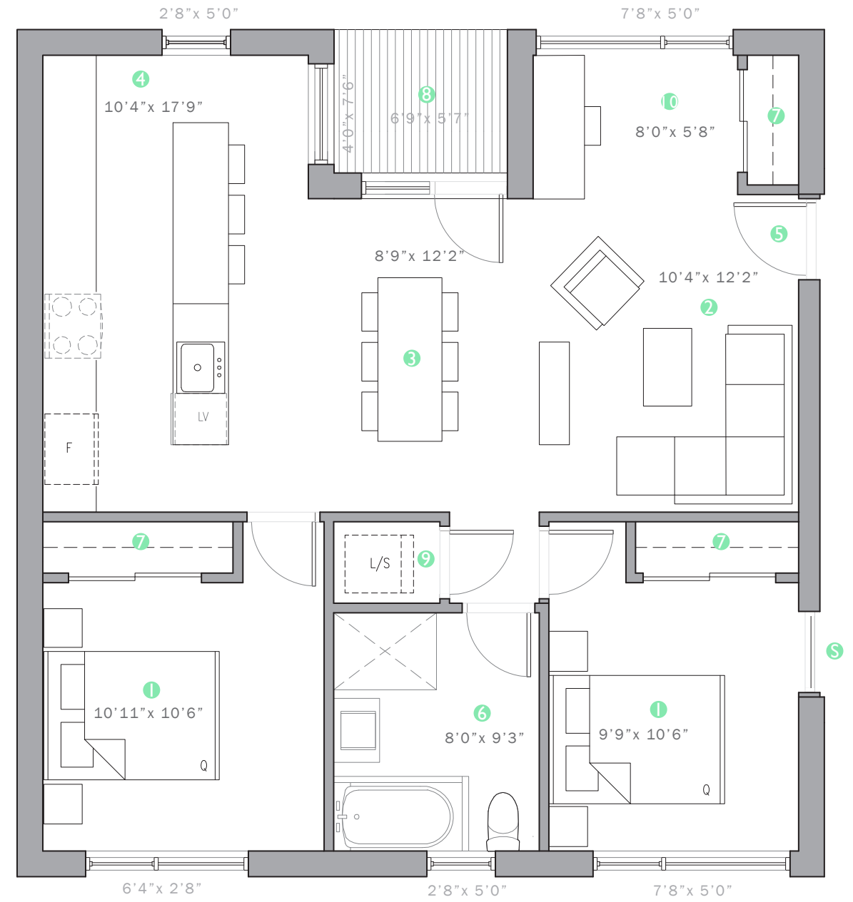
NIVEAU 1 (OPTION 2) - 996 PL.CA
