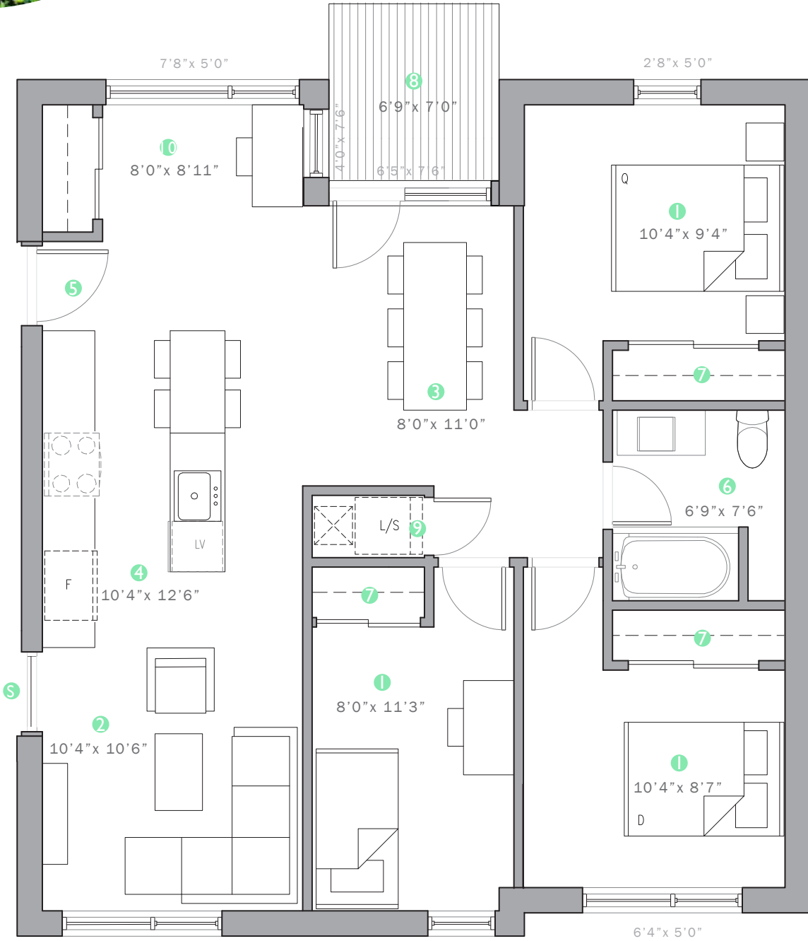
NIVEAU 2 (OPTION 1) - 1011 Pl.ca
